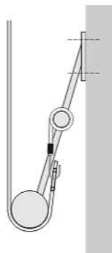
STRUTTURA CON TELAIO POSTERIORE
